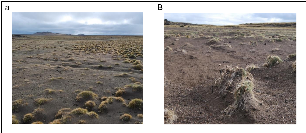
Figura 7. Área de acumulación de arena (a) y de erosión (b) asociada a una laguna temporaria.
